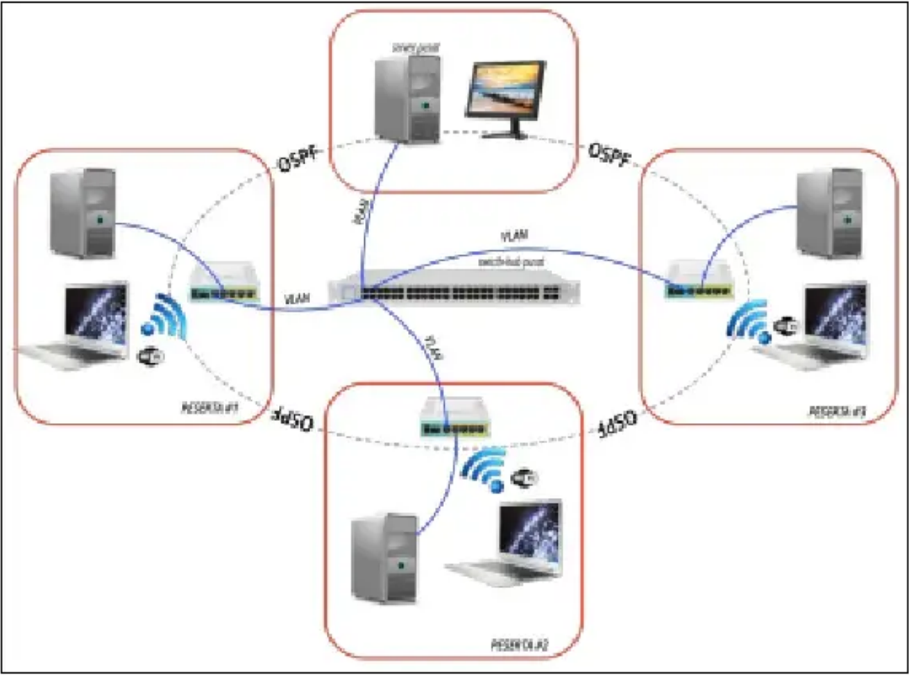
Gambar 1. Topologi jaringan untuk lomba.
